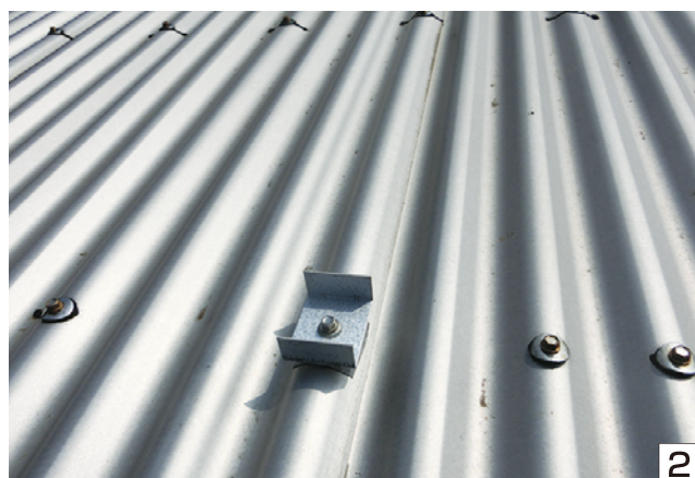
既設の大波ドリルスクリーブスを利用して コ型金具を取り付けます。
